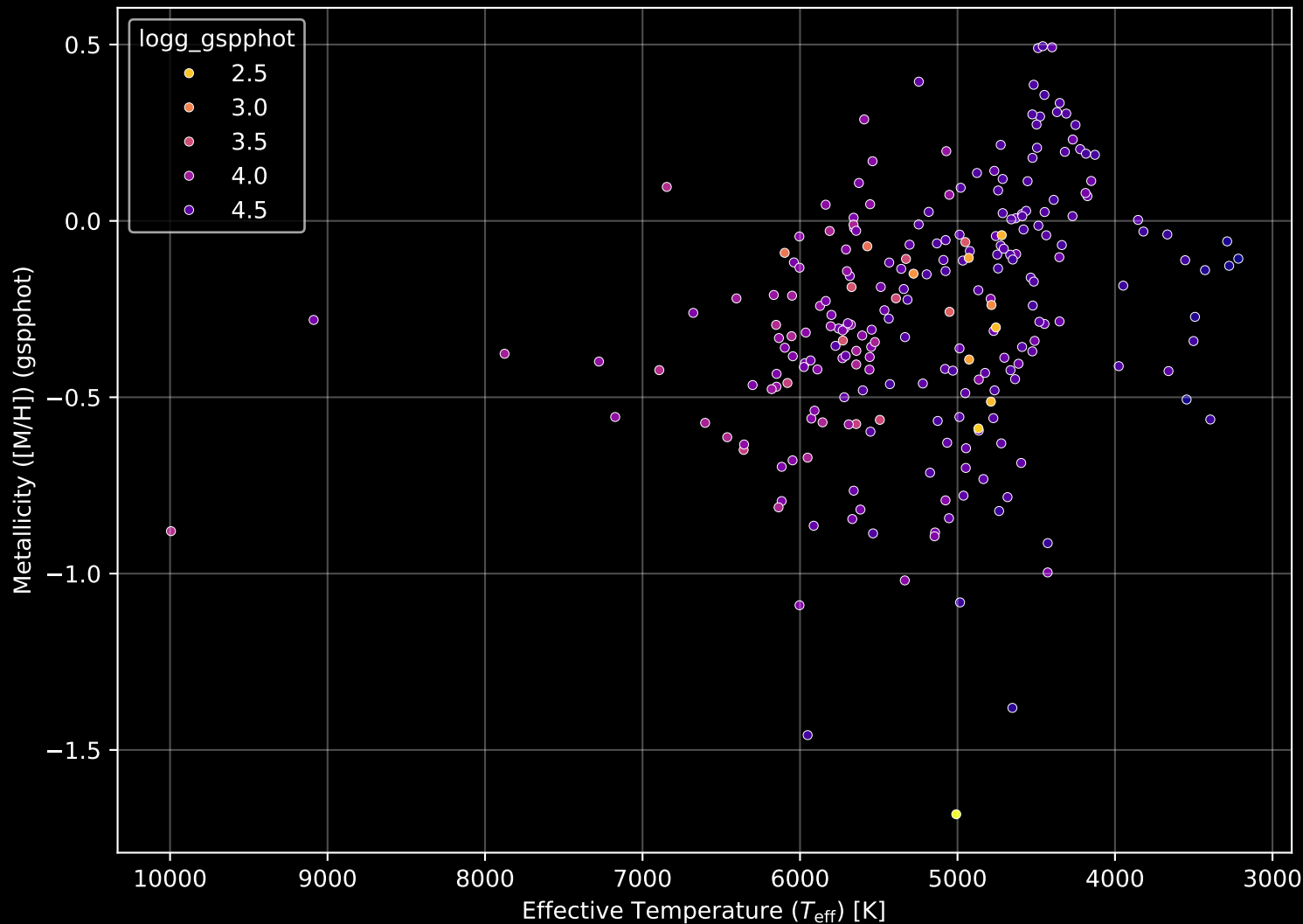
APOGEE DR17 Field: [K2_C12_065-59_btx] Stellar Population Parameters (n= 240)
